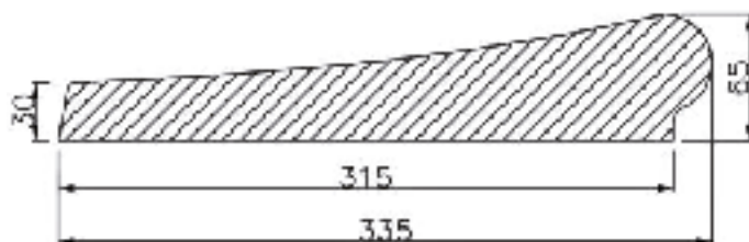
Disegno tecnico
